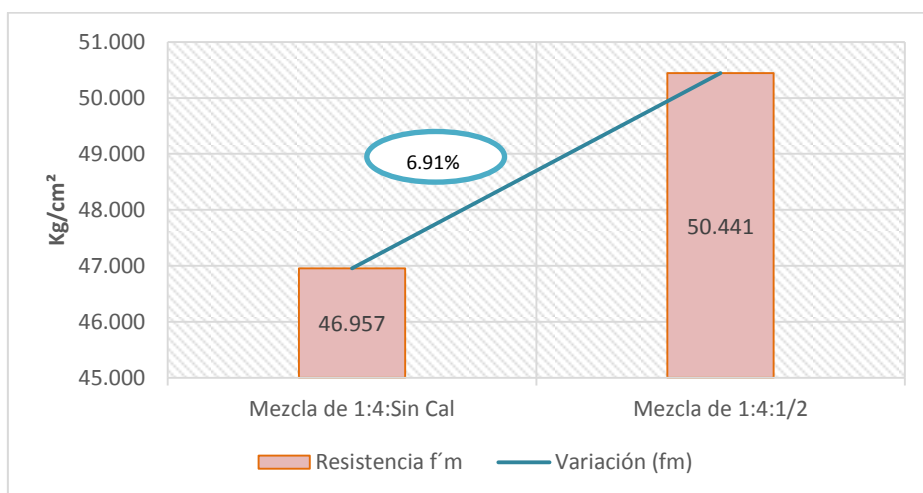
Figura 43. Resistencia f'm de pilas de ladrillo de arcilla industrial de 1:4 y 1:4:1/2
