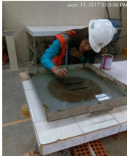
Figura 32. Ensayo de succión
