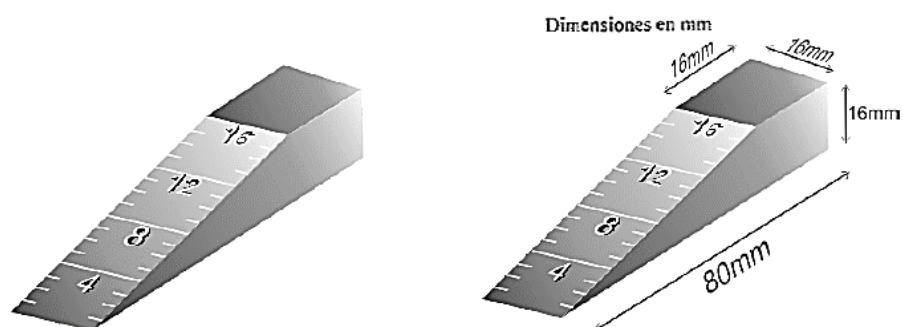
Figura 12. Cuña para medir el alabeo
