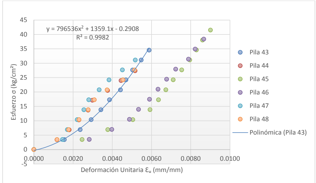
Figura 95. Esfuerzo vs Deformación unitaria (concreto artesanal de 1:5: 1/2)
