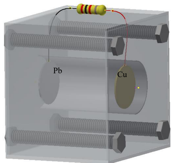
Fig. 1: Esquema del prototipo de las CCMs.
