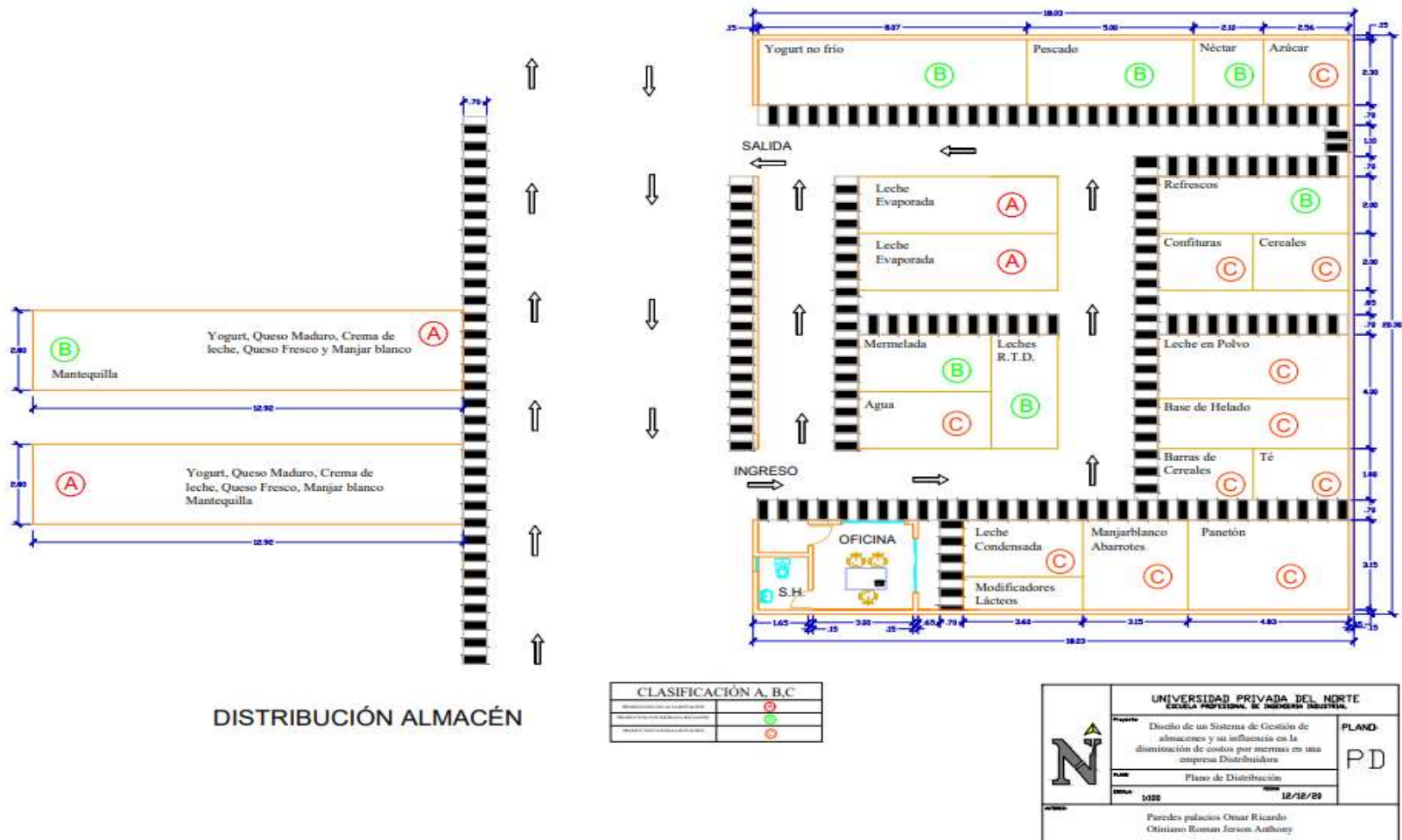
Figura 14 Layout de distribución
