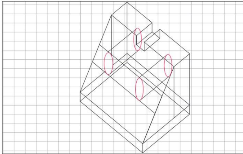
Fig. 5: Modelamiento en Civil 3D del muro que soportará la fuerza del caudal de las venidas de agua de la Quebrada San Idelfonso
