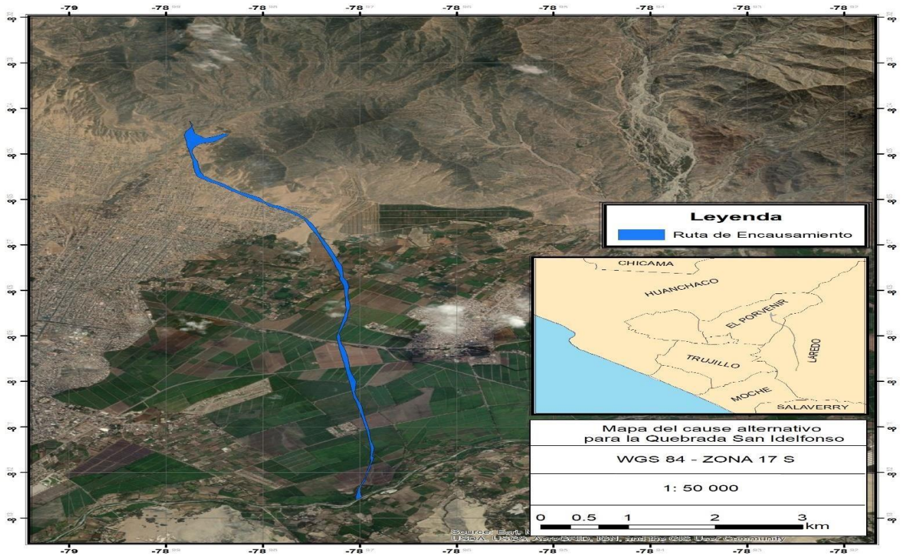
Fig. 6: Mapa de encausamiento de canal como alternativa de Solución.
