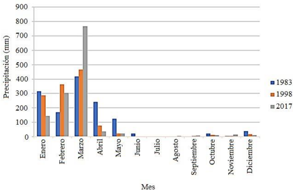
Fig. 2: Variabilidad pluviométrica mensual de los tres últimos Fenómenos del Niños acontecidos en la Quebrada San Idelfonso, en los últimos cincuenta años
