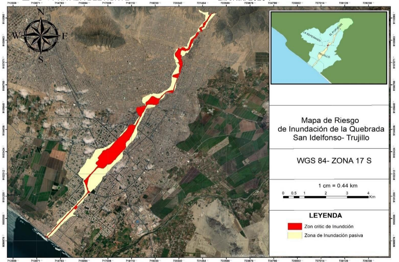
Fig. 4: Mapa de Riesgo y peligros de inundación de la Quebrada San Idelfonso
