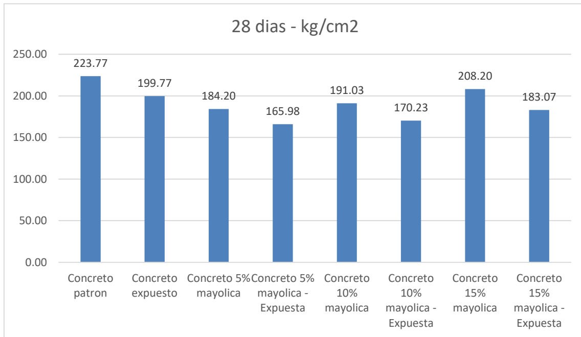
Resistencia a la compresión en 28 días
