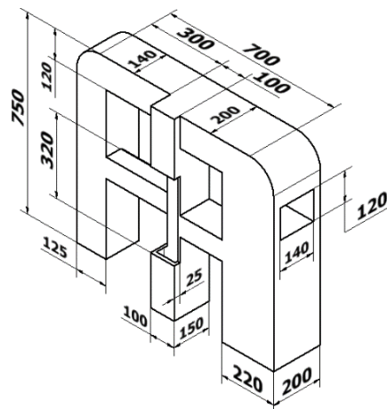
Fig. 11 Plano pieza 2: base izquierda.
