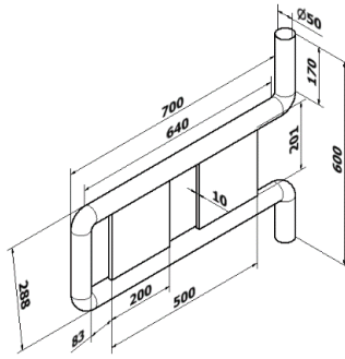
Fig. 12 Plano pieza 3: barrera oscilante.
