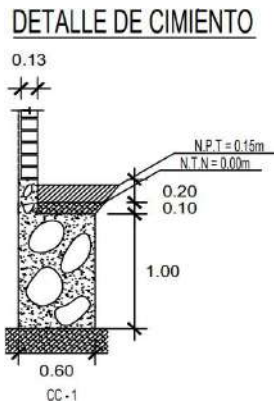
Fig. 14 Detalle del cimiento corrido (CC-1).
