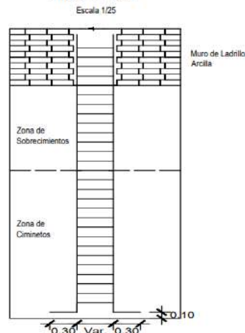
Fig. 9 Anclaje de columnas entre los muros.
