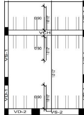
Fig. 12 Detalle de la Losa.
