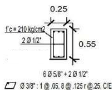
Fig. 15 Corte de la viga de cimentación con su acero respectivo.
