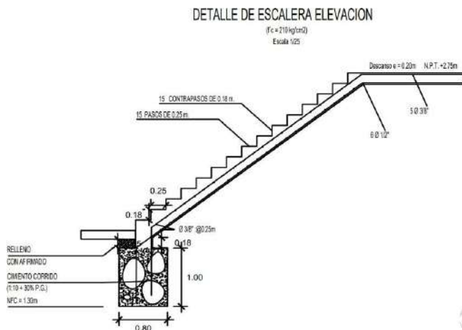
Fig. 11 Detalle de la escalera de elevación.
