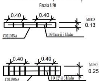
Fig. 7 Detalle de acero de refuerzo en los muros.
