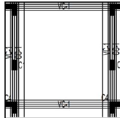
Fig. 13 Planta de la cimentación como el cimiento corrido y la viga de cimentación.
