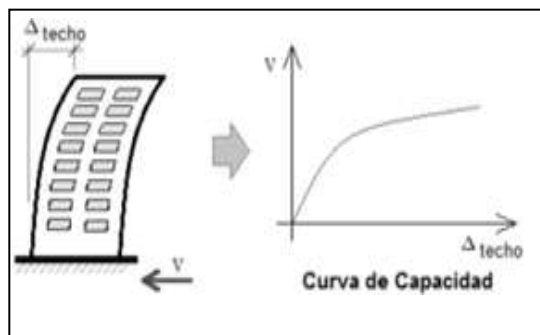
Fig. 1 Representación de la Curva de Capacidad.
