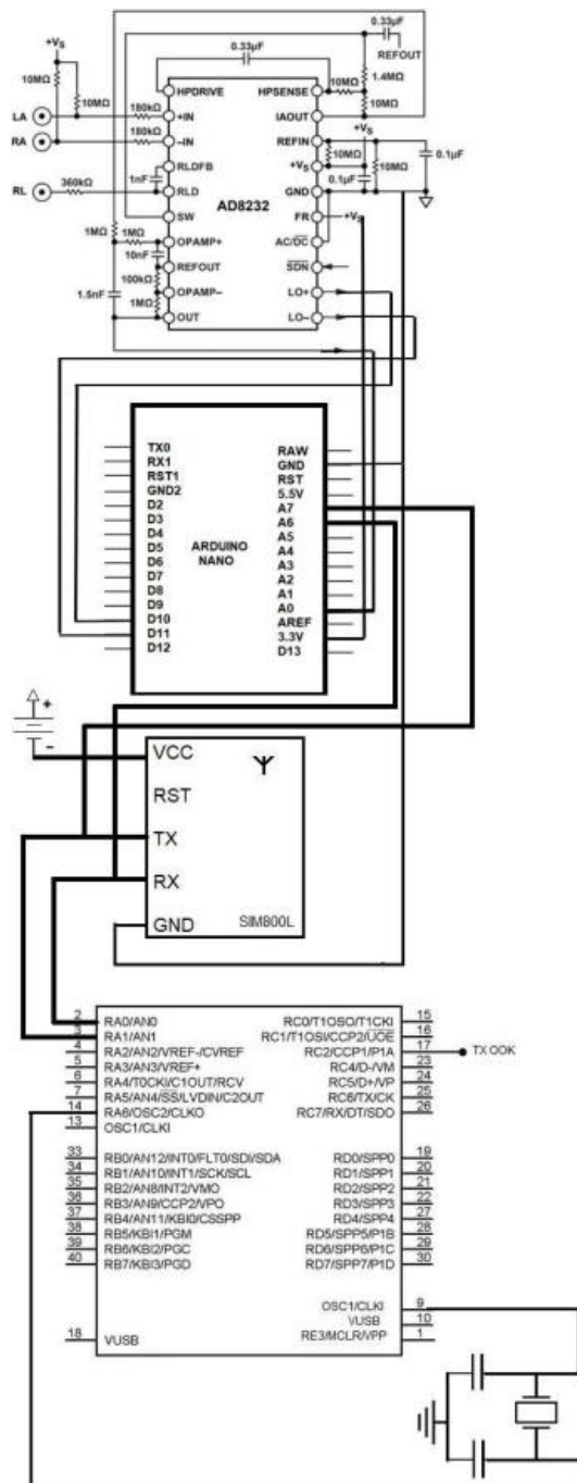
Fig. 2. Diagrama electrónico del electrocardiógrafo.
