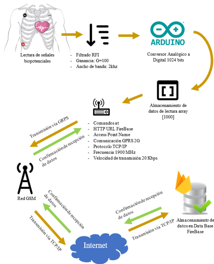
Fig. 3. Arquitectura del Electrocardiógrafo.
