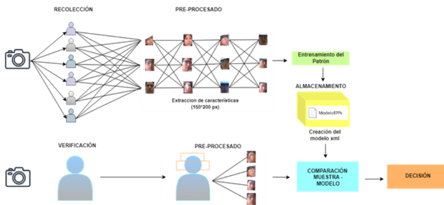
Fig.4 Arquitectura del algoritmo
