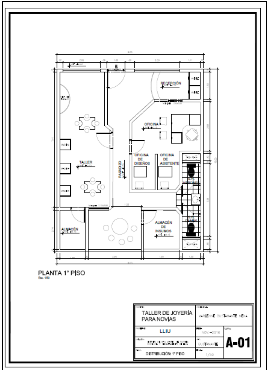
Figura N° 34. Plano de local de Oficinas y Taller de Producción
