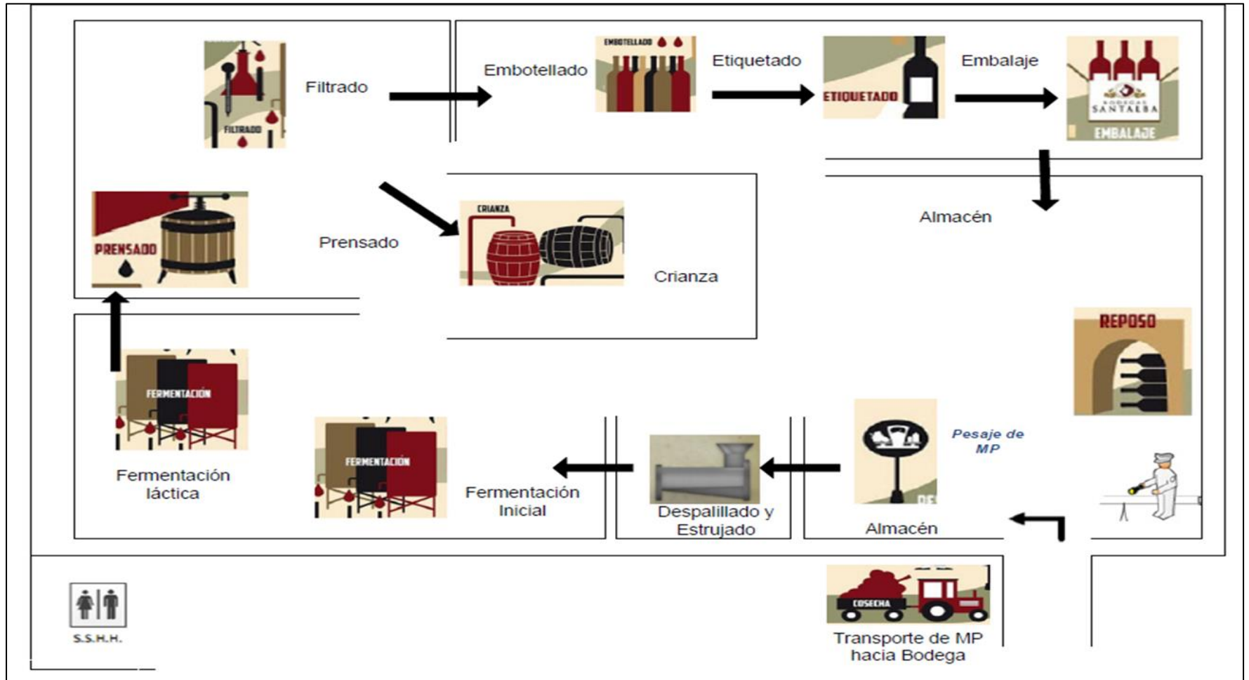
Gráfico N° 36: Distribución de Planta Propuesta - Bodegas El Zarco
