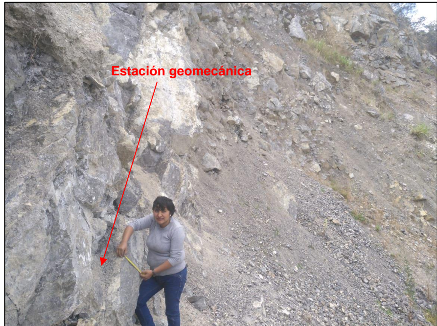
Figura 10. Estación geomecánica de la concesión San Juan.
