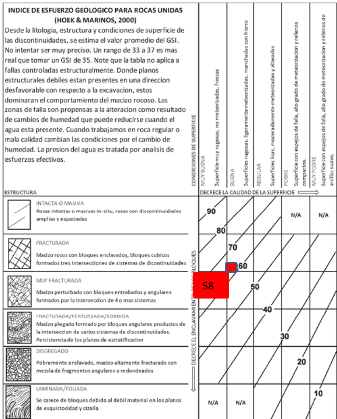
Figura 13: Clasificación geomecánica GSI.
