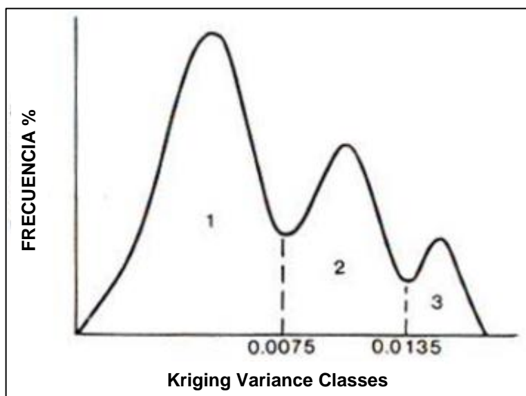
Figura 2: Histograma de las varianzas kriging ( V_k ) en 3 poblaciones: 1) Reservas probables, 2) Reservas posibles 3) Reservas inferidas. Fuente: (Vega, 2013).
