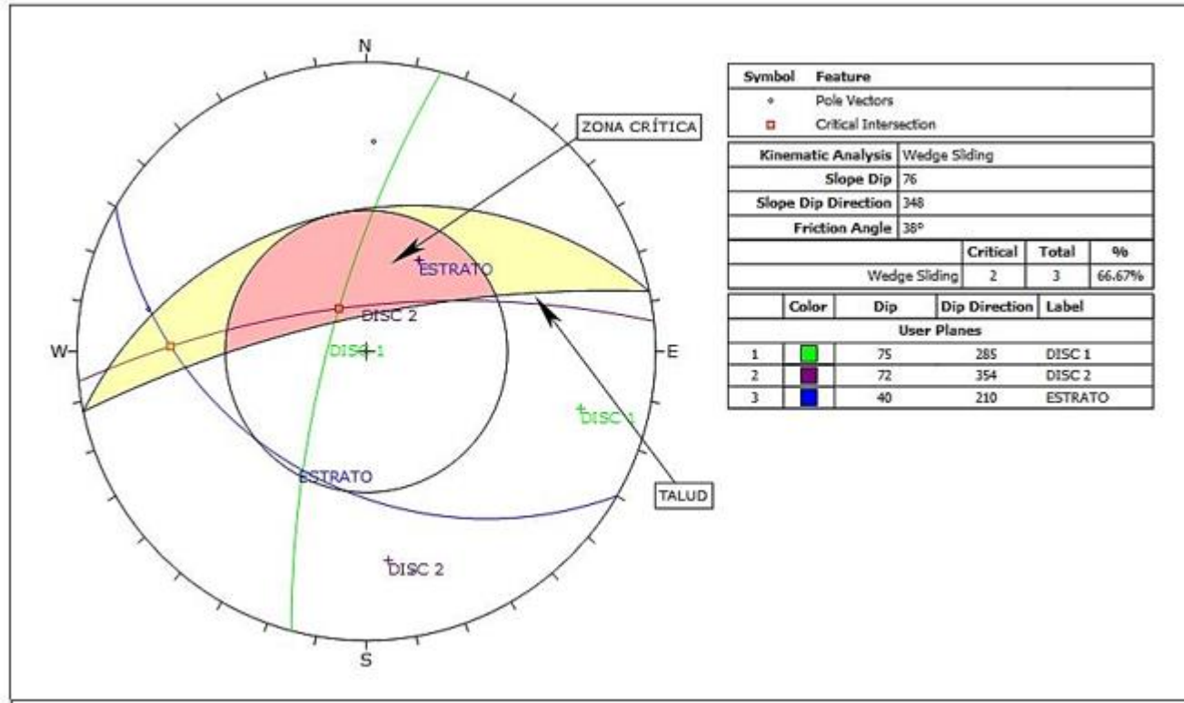
Figura 14. Diagrama de proyección estereográfica respecto al talud.
