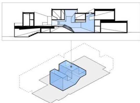
Figura 11 Corte longitudinal
