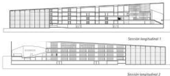
Figura 23 Corte longitudinal
