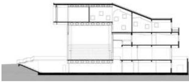
Figura 7 Corte transversal
