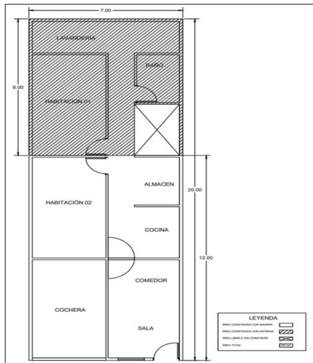
Figura 2: Vivienda de 7.00 x 20.00 m.
