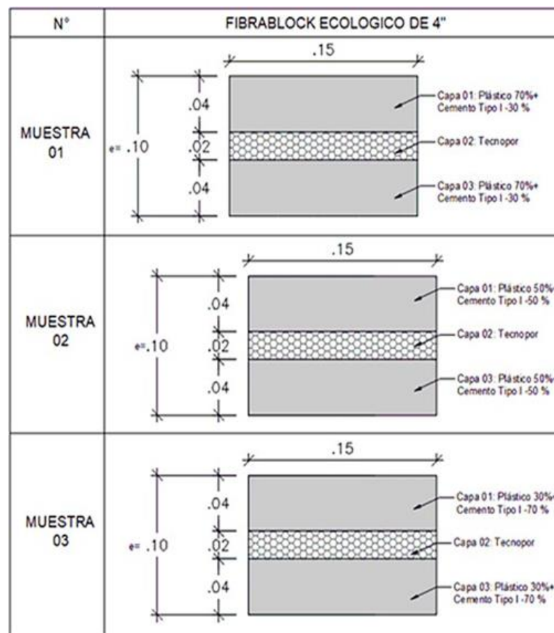
Figura 3: Muestras de moldes de 15x15x10 cm.
