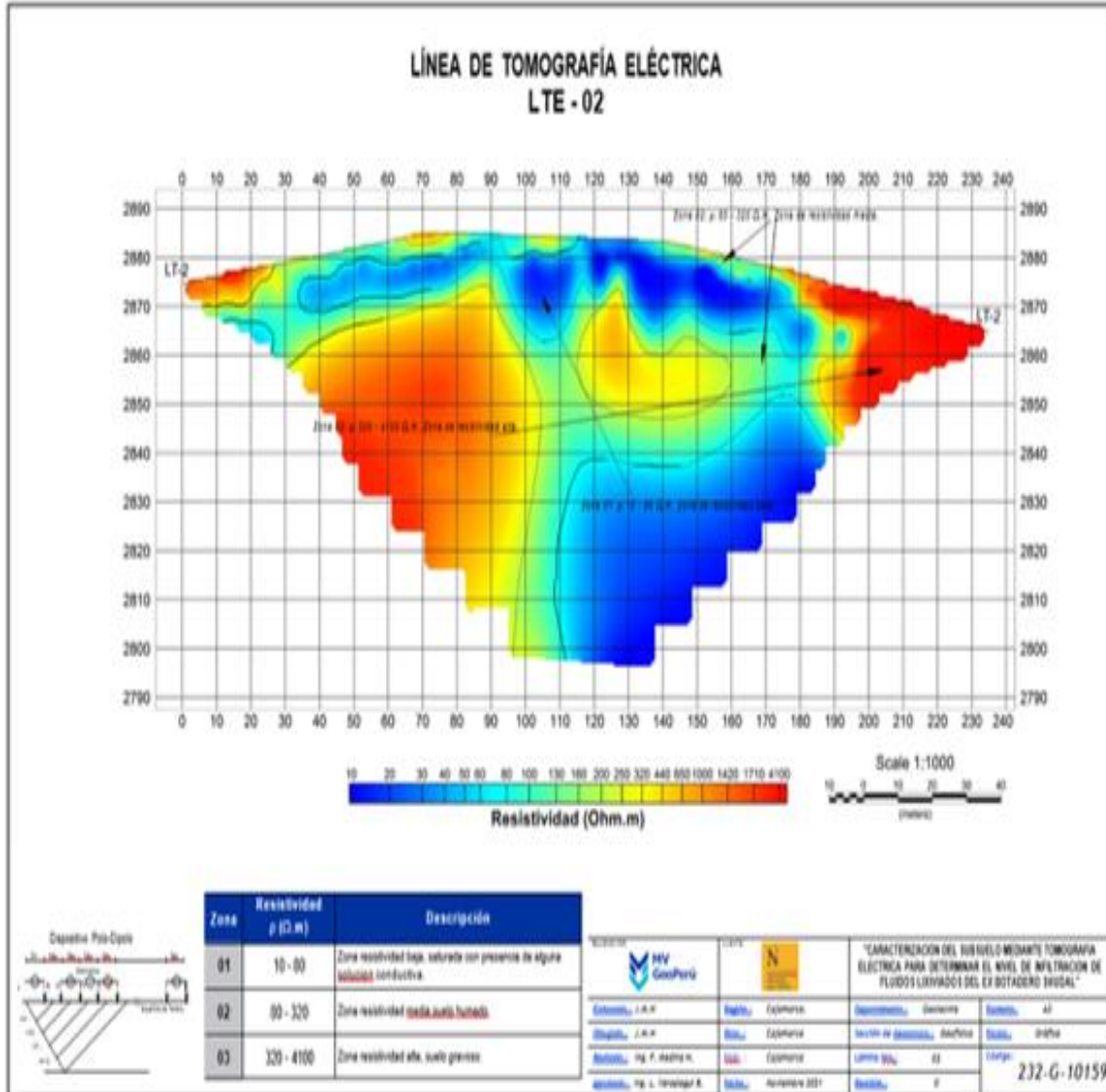
Ilustración 5. Perfil de resistividades LTE - 02
