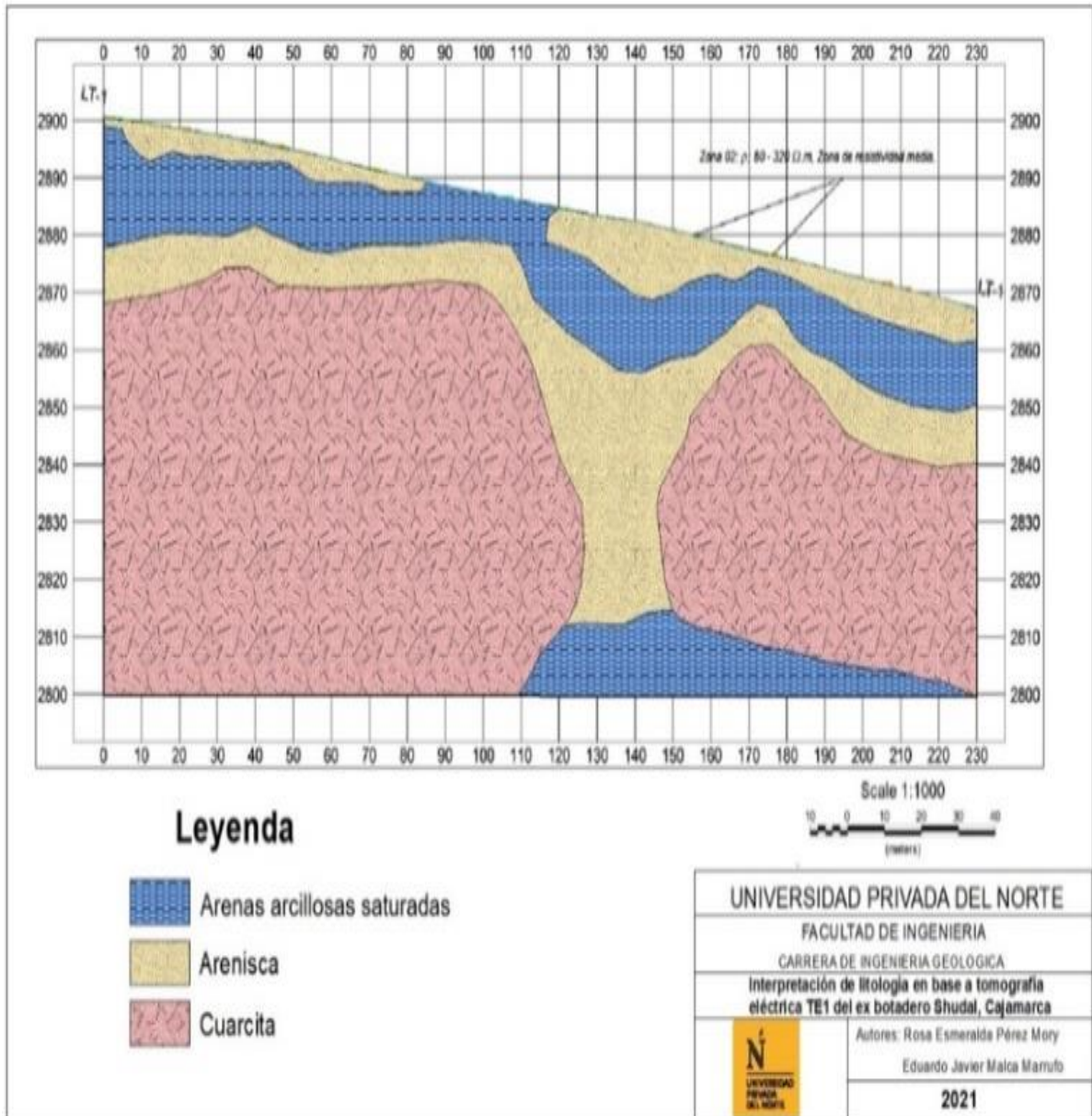
Figura 6. Interpretación litológica LTE - 01
