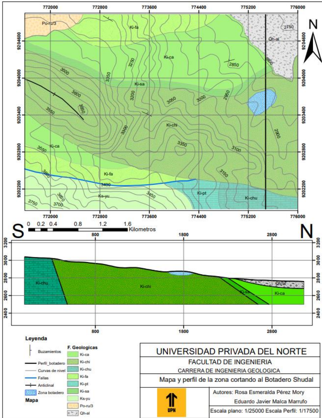
Ilustración 2. Geología de la zona
