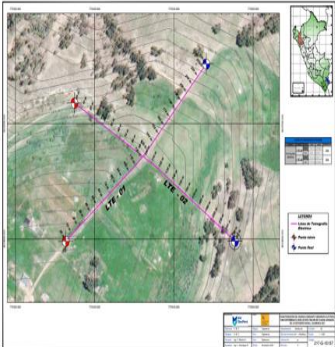
Ilustración 3. Plano topográfico y líneas referenciales a las tomografías de la zona
