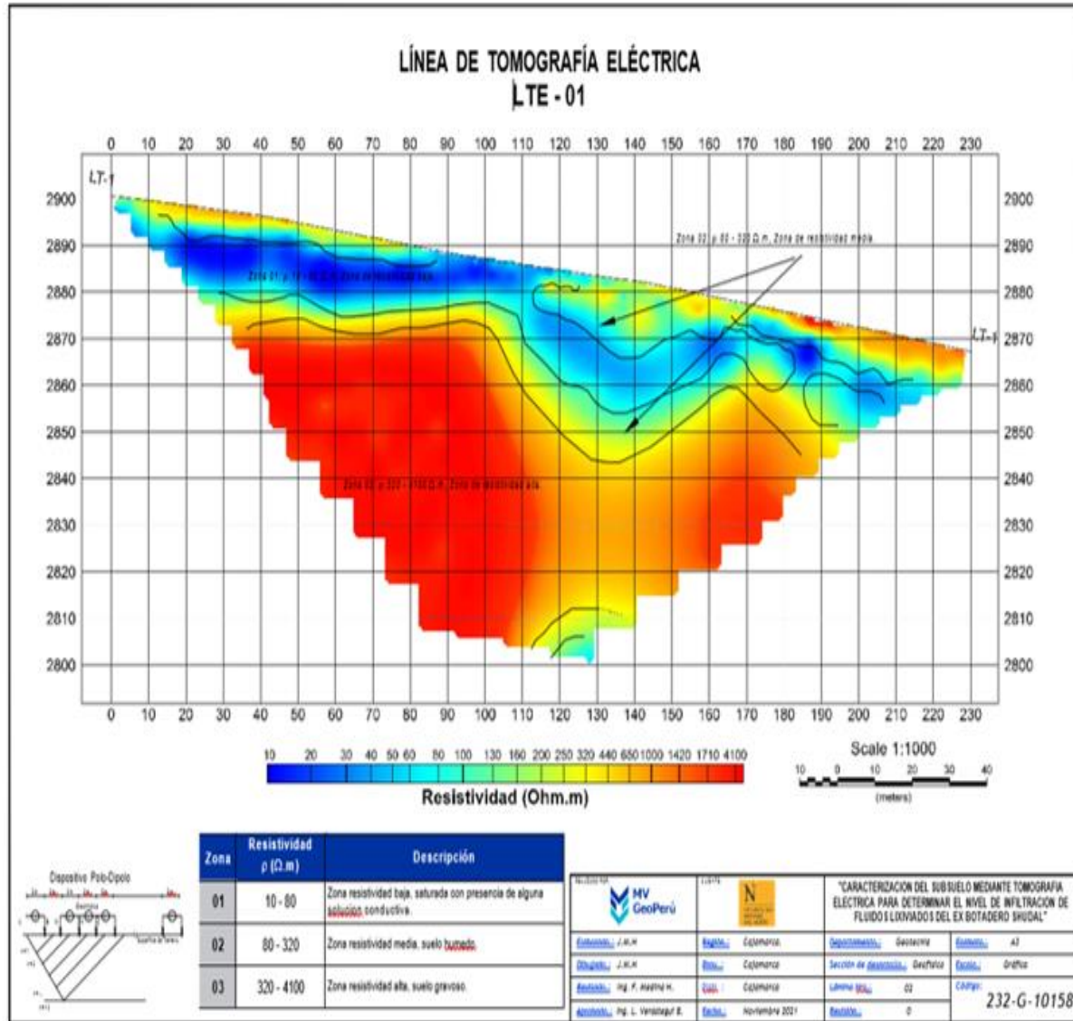
Ilustración 4. Perfil de resistividades LTE - 01
