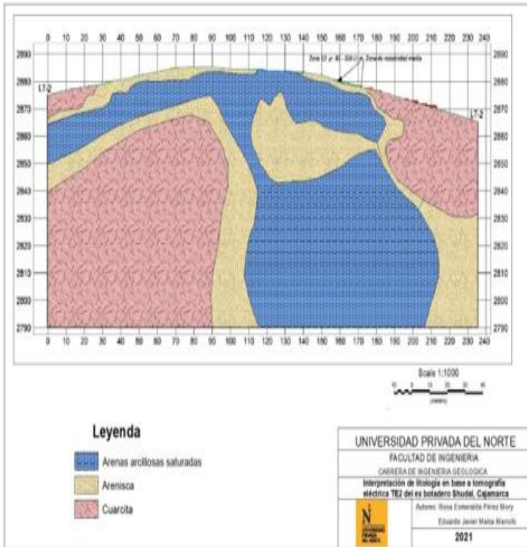
Figura 7. Interpretación litológica LTE - 02
