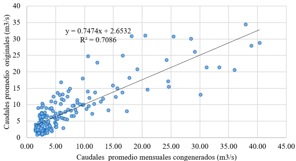
Figura 10 Curva de calibración entre caudales promedio mensuales generados con el método GR4j y caudales registrados para la cuenca del río Zaña hasta la estación hidrométrica Batán (01/2000 - 11/2015).
