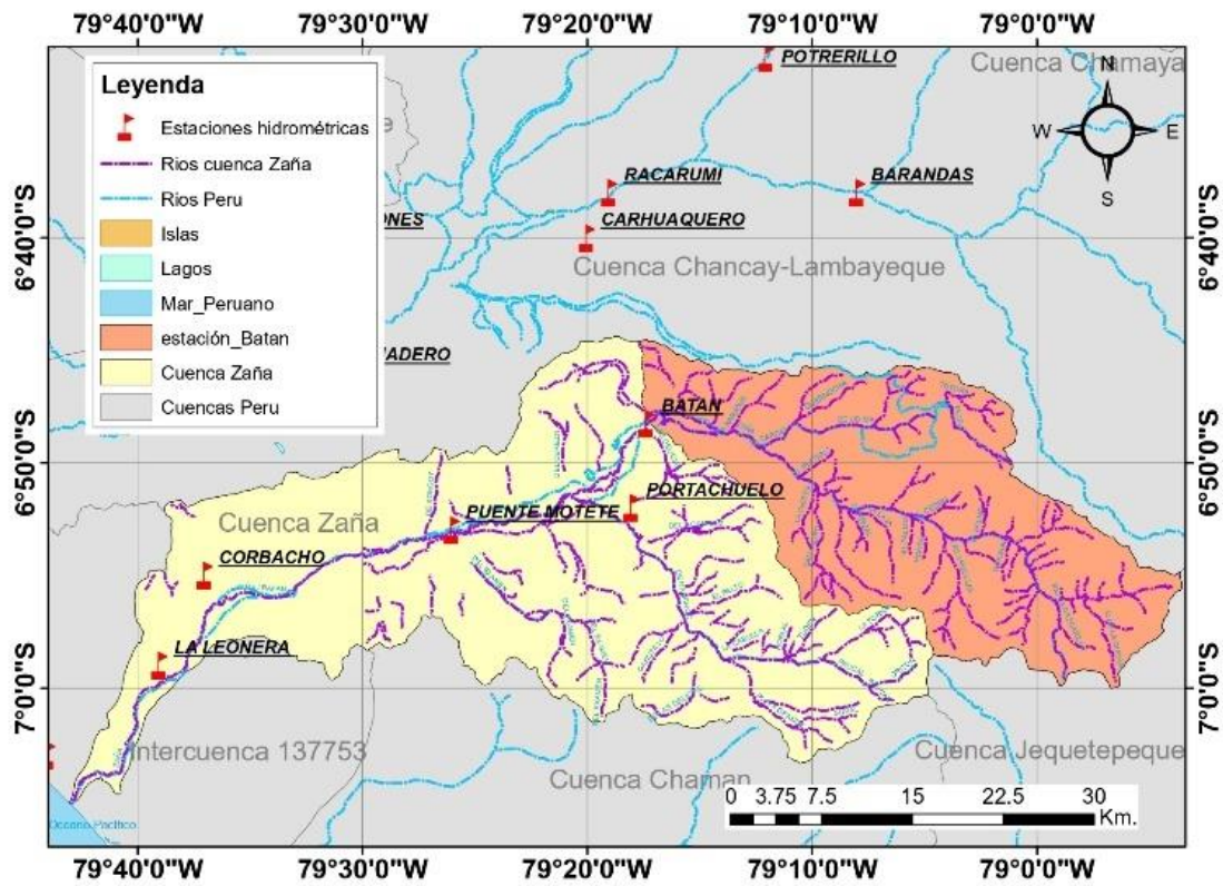
Figura 11 Delimitación de la cuenca Zaña completa y hasta su cierre en la estación hidrométrica Batan.
