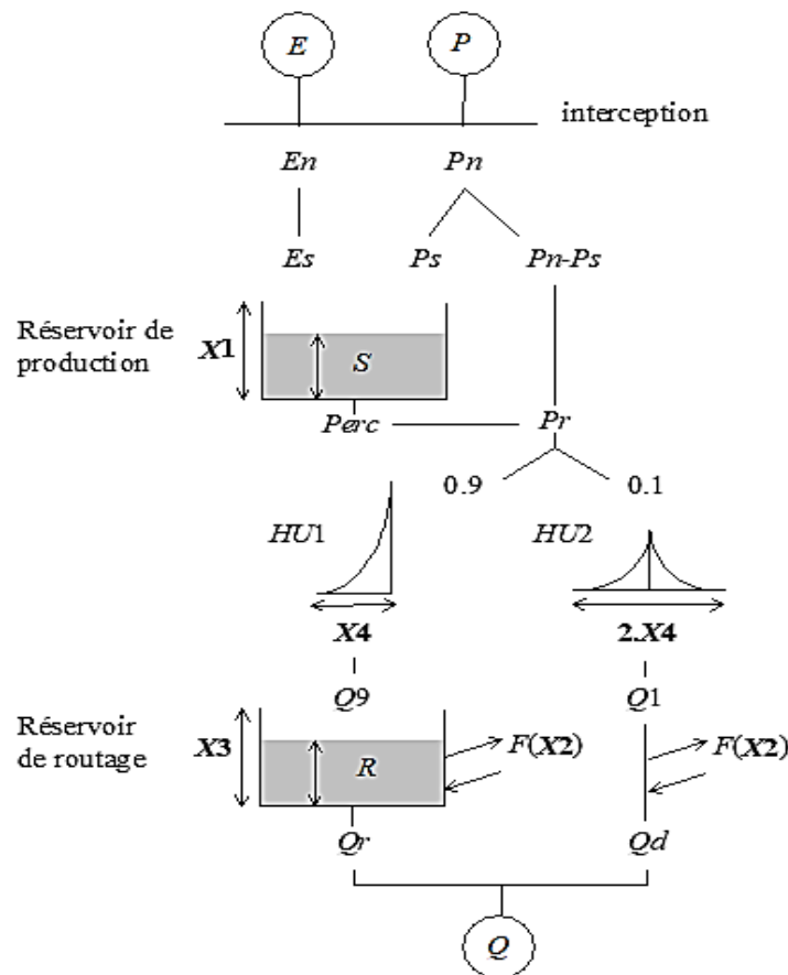
Figura 1 Modelo hidrológico GR4J. Fuente: Carvajal, L. y Roldán, E. (2007)
