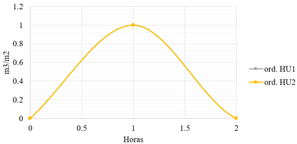
Figura 8 Hidrogramas unitarios para la etapa de validación.
