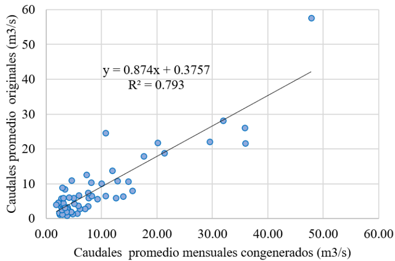
Figura 6 Curva de calibración entre caudales promedio mensuales generados con el método GR4j y caudales registrados para la cuenca del río Zaña hasta la estación hidrométrica Batán (1/12/2015 - 8/7/2020).
