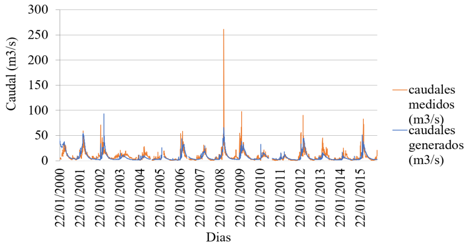
Figura 9 Comparación entre caudales diarios medidos y los caudales generados con datos de precipitación de ERA5 y el método GR4j para la cuenca del río Zaña hasta la estación hidrométrica Batán (01/01/2000 - 30/11/2015).
