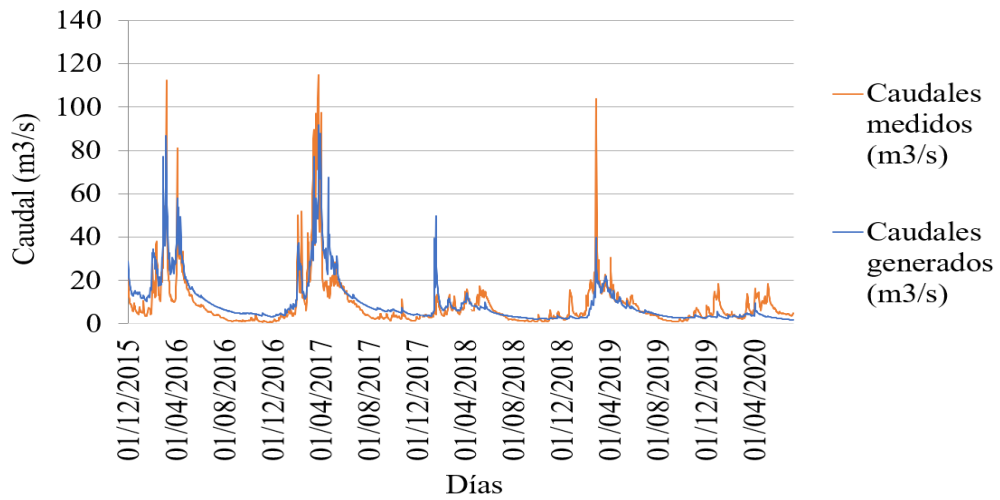
Figura 5 Comparación entre caudales diarios medidos y los caudales generados con datos de precipitación de ERAS5 y el método GR4j para la cuenca del río Zaña hasta la estación hidrométrica Batán (1/12/2015 - 8/7/2020).
