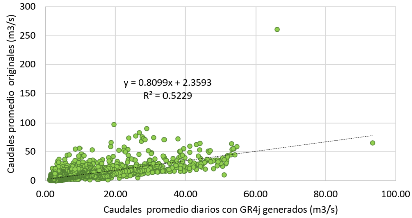
Figura 7 Correlación entre caudales observados y caudales generados por el modelo en la etapa de validación.
