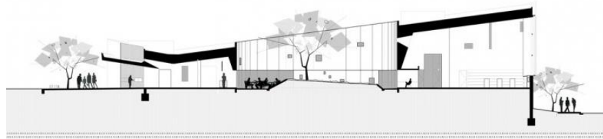
GRÁFICO N° 13. Corte transversal de la Biblioteca de Hércules.
